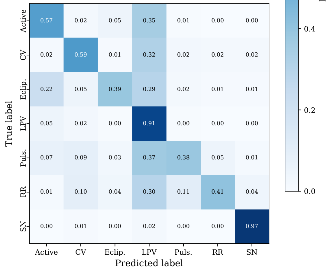
(d) E2E Transformer (no pre-training)
